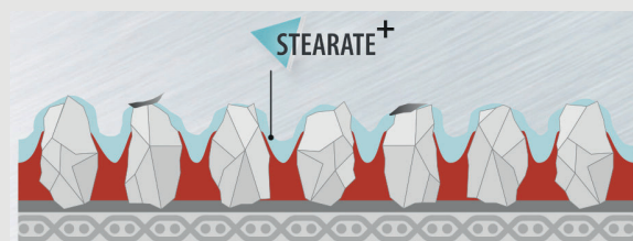
Die Zusatzschicht VSM STEARAT Plus verringert deutlich das Anhaften, das Schleifmittel kann länger genutzt werden.
