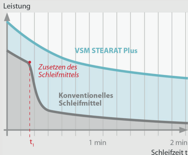
Schleifen von Stangenmaterial ( \varnothing 30 mm) aus Aluminiumlegierung (AlSi12Cu) mit Fiberscheiben in Korngröße 24.
