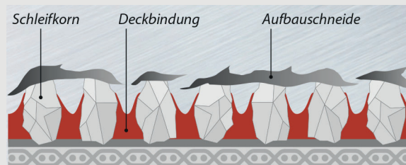
Konventionelles Schleifmittel: Späne bleiben an den kornspitzen haften, das Schleifmittel setzt sich zu.
